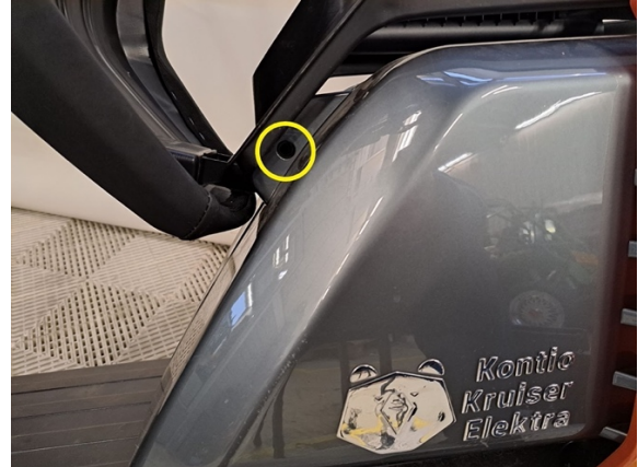
Irrota vasenta kylkipaneelia kiinnittävä ruuvi (ristipäämeisseli ph2).
