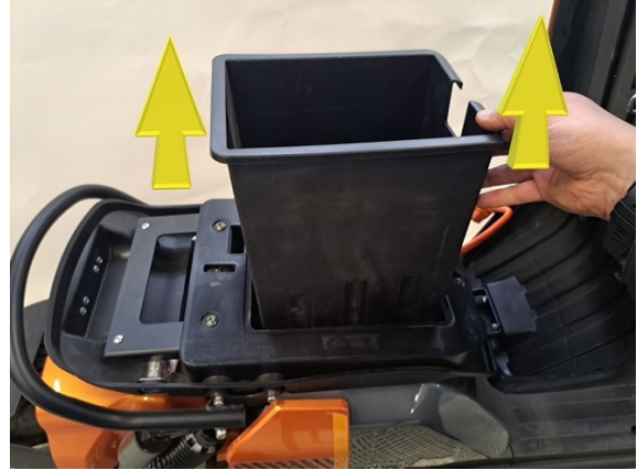
Nosta akkulaatikko pois.
