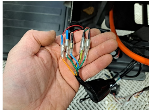
Avaa takavoille menevät liittimet.
