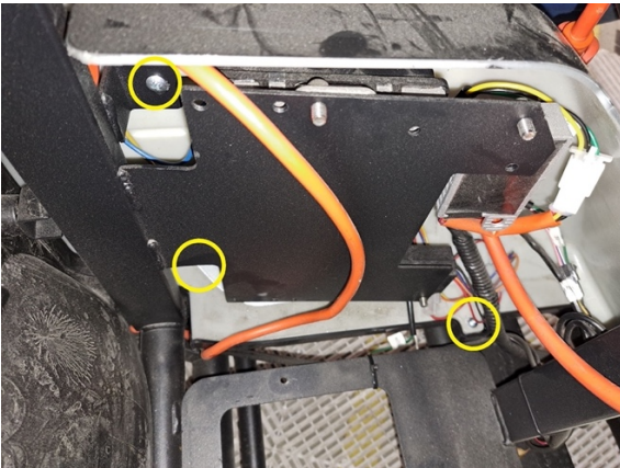
Irrota vasemmanpuoleisen kylkipaneelia kolme kiinnitysruuvia. (Ristipäämeisseli ph2).
